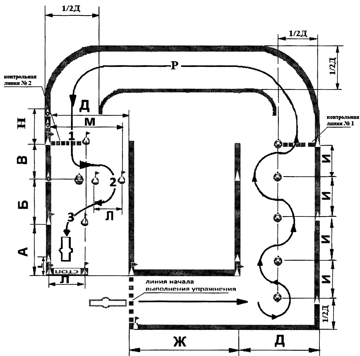
Схема "Б" элемента упражнения N 1 - "Скоростное маневрирование".
