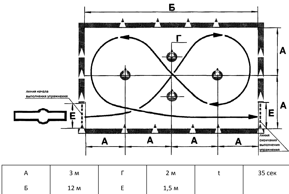
Рисунок 1. Схема и размеры элемента упражнения N 1 - "Габаритная восьмерка"
